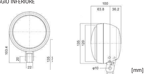
MONTAGGIO INFERIORE
