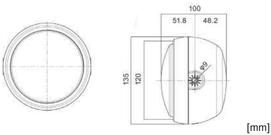
MONTAGGIO LATERALE
