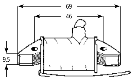
00.1636 Impianto Ducati Energia - uscita cavo lat. dx
