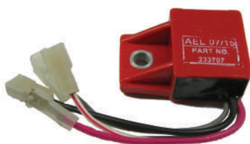
1233707 Dispositivo antiripetitore avviamento Vespa PX 125-150-200-30 anni Vespa T5
