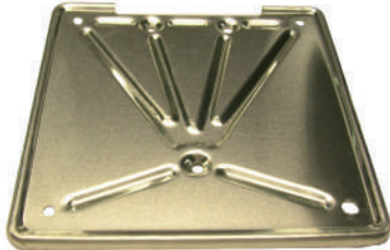
62073 Supporto targa Vespa 150 GS - 160 GS - P. 24667
