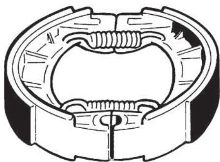
55098 Coppia ganasce - Grimeca mozzo ø 140
