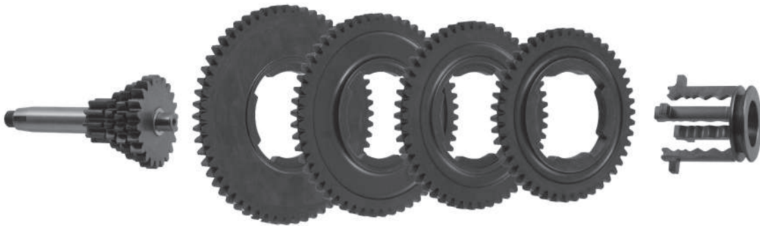
71000 SA Gruppo cambio - Vespa 50 - 4 velocità
