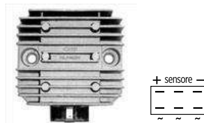
17.2064 regolatore DZE 12V - trifase - c.c. - 6 faston - c/sensore
