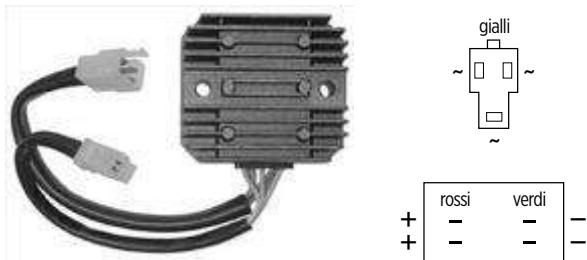
17.2061 regolatore DZE 12V - trifase - c.c. - 7 cavi - 2 connettori
