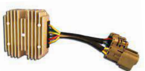
17.9160 regolatore 12V/35A - c.c. - trifase - 6 cavi - c/2 connettori grigi
