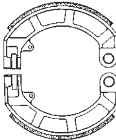
◀ cod. CP00210 Coppia ceppi Ø 150x24 Piaggio Vespa
