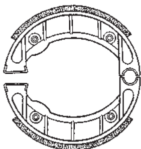
◀ cod. CP00201 Coppia ceppi Ø 105 x 20 con molle
