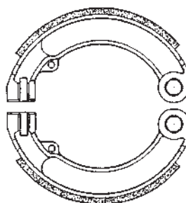
◀ cod. CP00211 Coppia ceppi Ø 125x19 Piaggio Vespa
