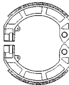
◀ cod. CP00212 Coppia ceppi Ø 150 x 24 Piaggio Vespa PX - PK anteriore e posteriore
