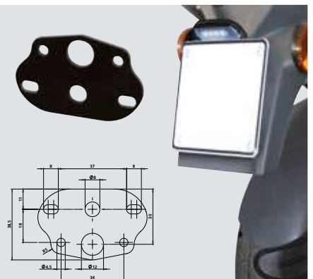
SUPPORTO LUCE TARGA PER CICLOMOTORI In alluminio. Peso 13 g Finitura a polvere epossidica.
