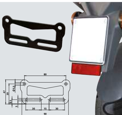
SUPPORTO PER CATARIFRANGENTE TARGA CICLOMOTORI In alluminio. Finitura a polvere epossidica. Peso 20 g
