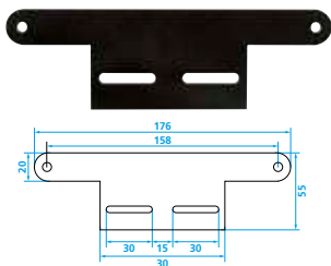
SUPPORTO PER CATARIFRANGENTE TARGA In alluminio anodizzato. Asole di fissaggio.
