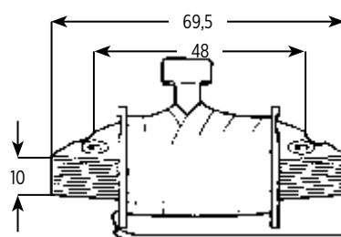
00.1107 impianto Filso
