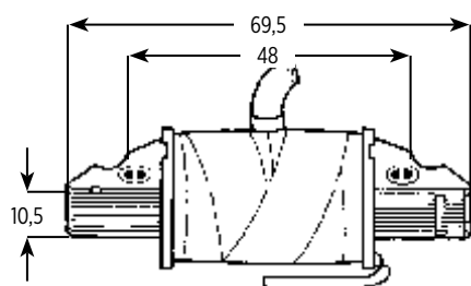
00.1136 impianto CEV
